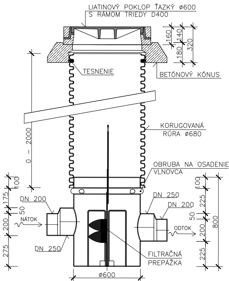
Rez č.1 s predĺžením a poklopom D400
