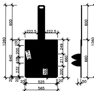
Filtračná prepážka do FŠ600
