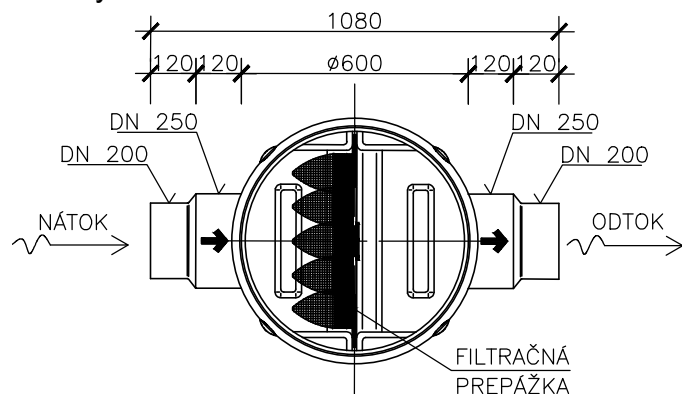
Filtračná prepážka do FŠ600
