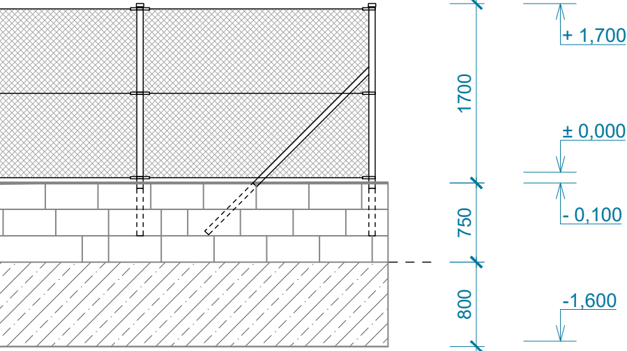
Oplotenie vyrovnávajúce výškový rozdiel terénu
