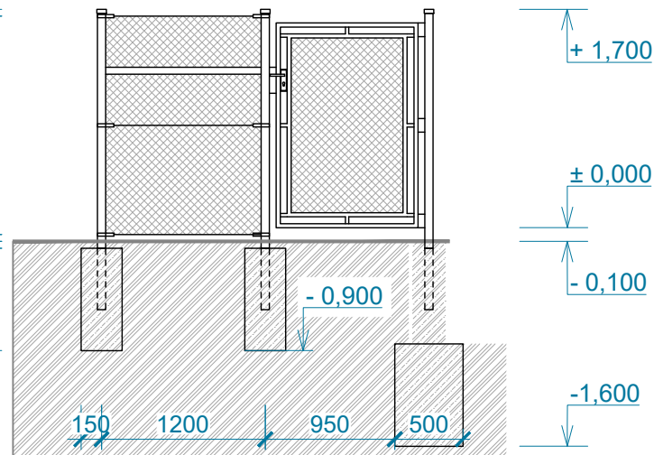
Oplotenie vyrovnávajúce výškový rozdiel terénu - oporný múrik
